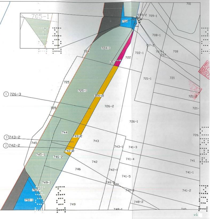
彰化縣新街海堤堤段整建工程 (0K+000-1K+000、2K+700-3K+716) 用地範圍圖說(2/8) (都市土地)
