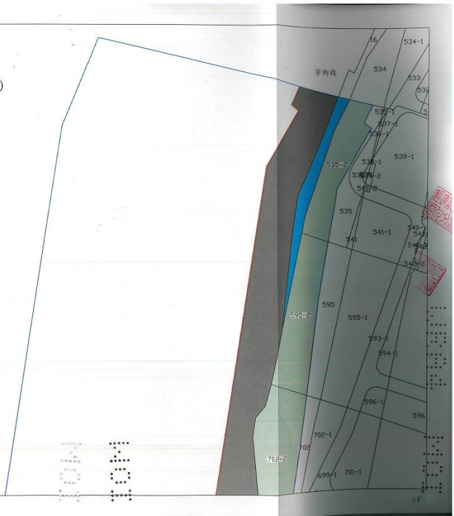
彰化縣新街海堤段整建工程 (0K+000~1K+000、2K+700~3K+716) 用地範圍圖說(1/8)(都市土地)
