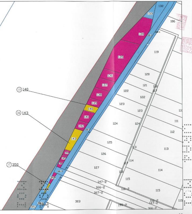
彰化縣新街海堤堤段整建工程 (0K+000-1K+000、2K+700-3K+716) 用地範圍圖說(6/8) (非都市土地)
